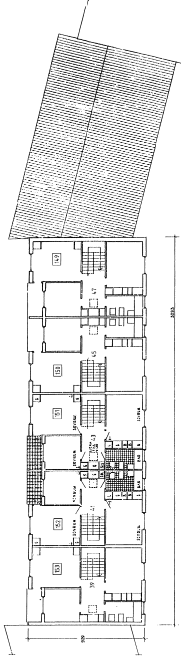
PLAN 1 TR. STARBOVÄGEN
